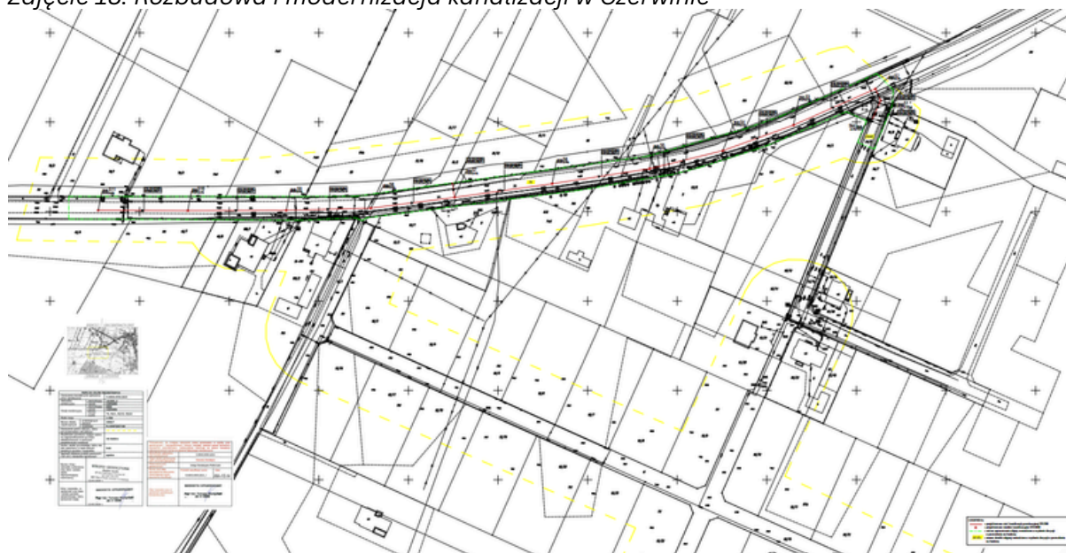
Zdjęcie 18. Rozbudowa i modernizacja kanalizacji w Czerwinie
